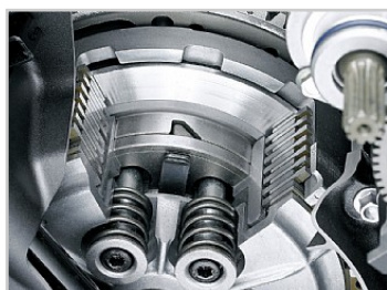
Verstelbare slijpkoppeling
