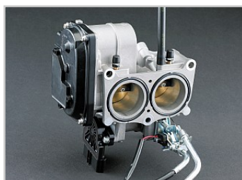
Elektronische gasklepsysteem (ETV)
